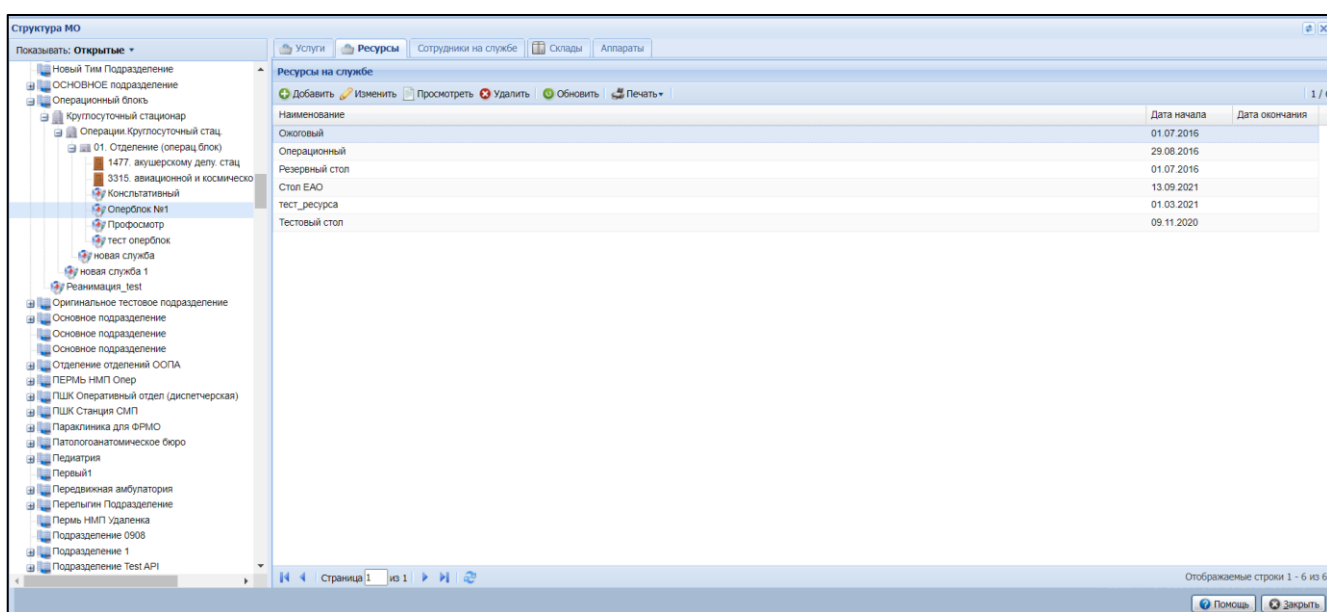
Рисунок 14 – Вкладка "Ресурсы"
